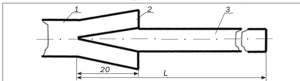
Рисунок 4.2 – Схема разделки ОК с бронепокровом из стальной гофрированной ленты 1 – наружная сталеполиэтиленовая оболочка; 2 – участок оболочки, симметрично разрезанный на 4 лепестка совместно со стальной гофрированной лентой; 3 – внутренняя оболочка
