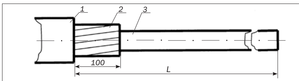
Рисунок 4.1 – Схема разделки ОК с бронепокровом из стальных оцинкованных проволок 1 – наружная полиэтиленовая оболочка; 2 – бронепокров из стальных оцинкованных проволок; 3 – внутренняя оболочка
