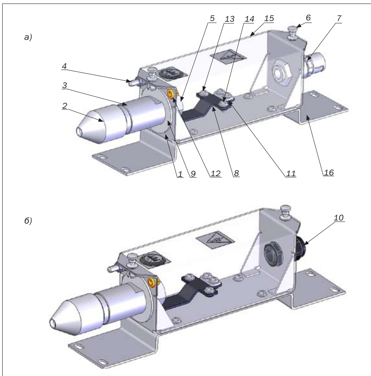
Рисунок 1.1 – Общий вид ВКУ-1 (а) и ВКУ-2 (б)
