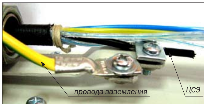
Рисунок 4.11 – Крепление на кронштейне ЦСЭ (металлический трос с полимерным покрытием) кабеля и провода заземления
